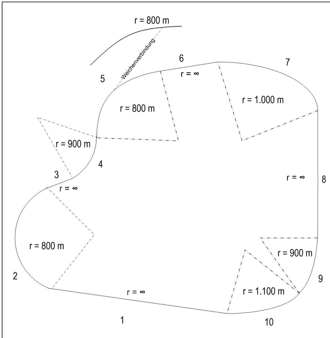
Abb. 1: Geplante Trassierung
